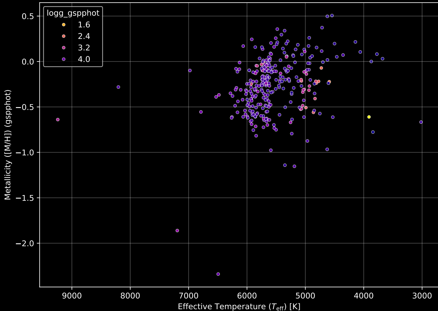
GALAH DR4 Field: [7011] Stellar Population Parameters (n= 305)
