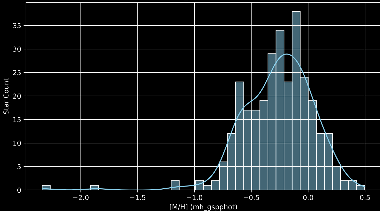
GALAH DR4 Field: [7011] [M/H] (mh_gspphot) (n= 304)
