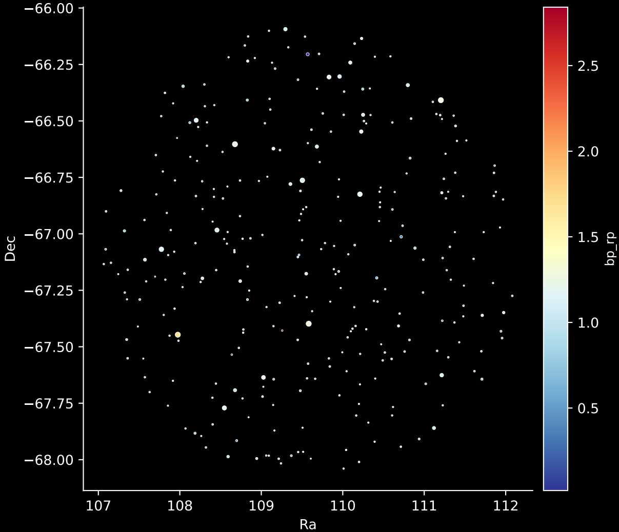
GALAH DR4 Field: [7011] Stars: 305
